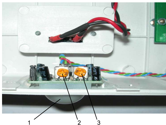
Рисунок 6.2. Расположение органов управления на плате датчика движения
