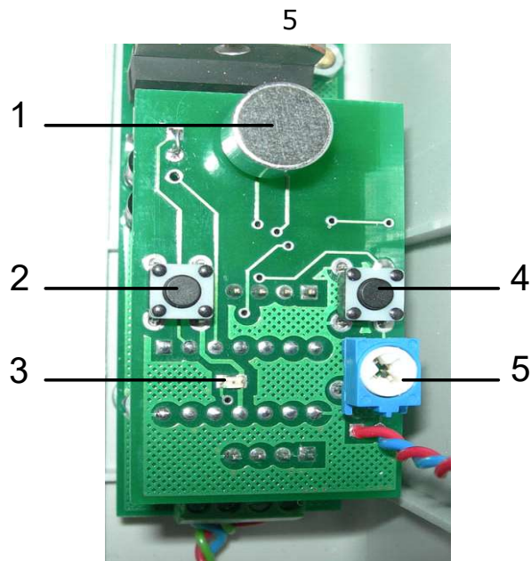
Рисунок 6.1. Расположение органов управления на плате диктофона
