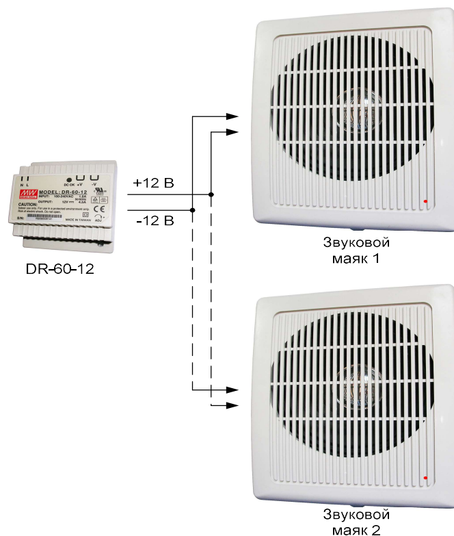
Рисунок 2.2. Структурная схема применения звукового маяка
