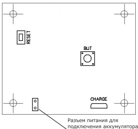
Рисунок 2. Внешний вид платы радиокнопки вызова MP-413W13
