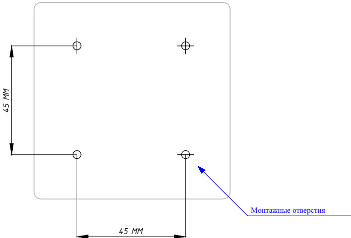
Кнопка GC-0421W1 и GC-0423W1 (задняя сторона)
